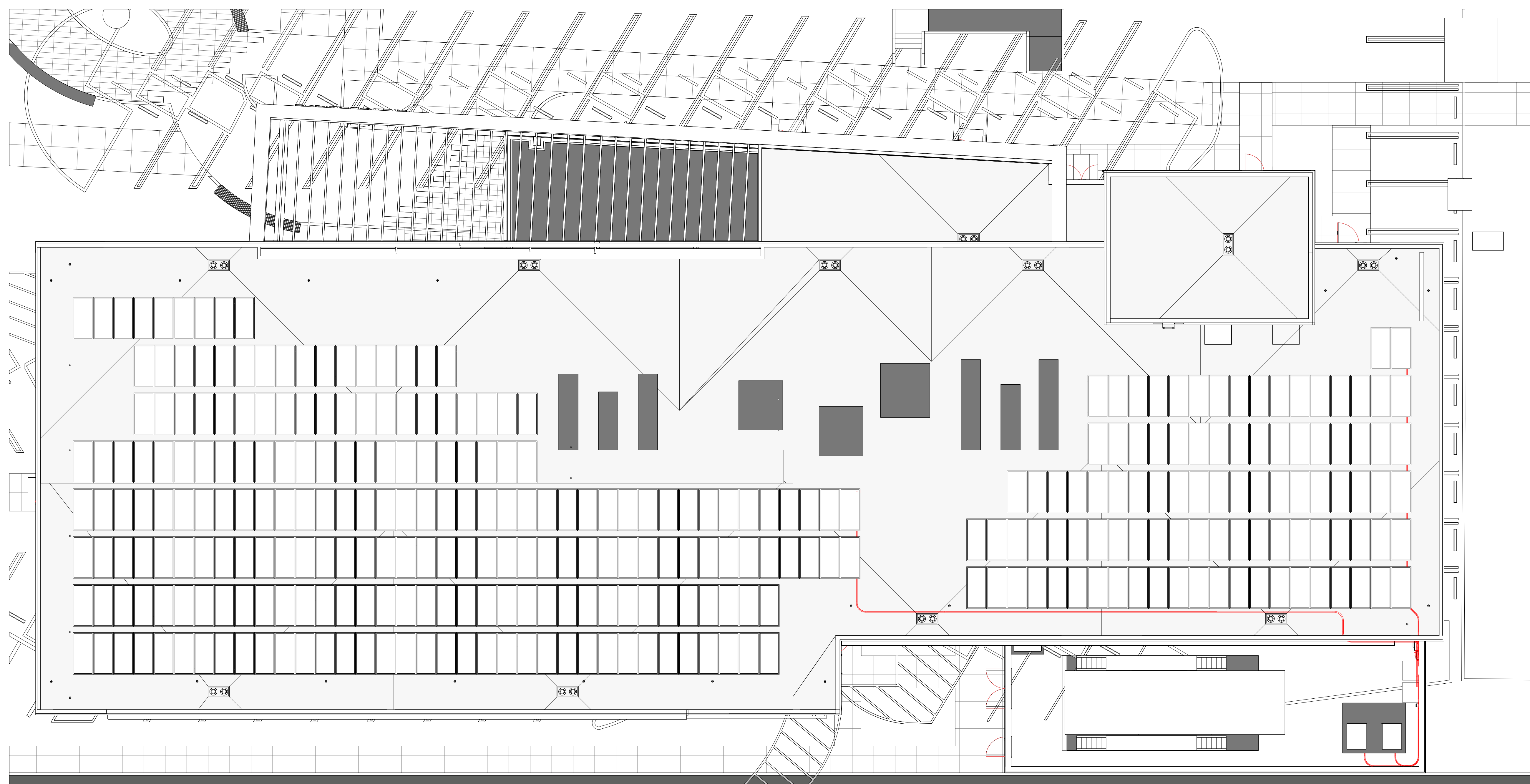
Solar Array PV conduit route
